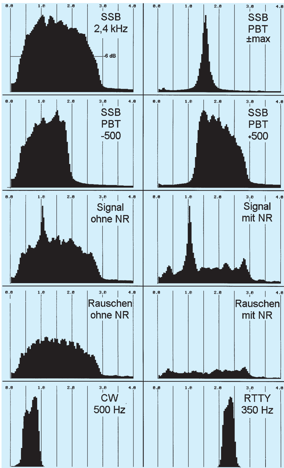
Bild E11: NF-Frequenzgang
